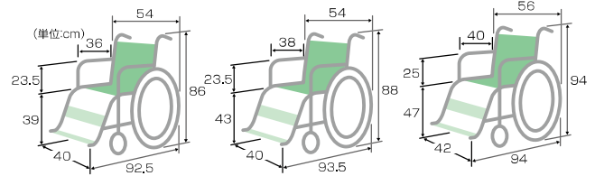
プチ NEXT-20B (低床型)
