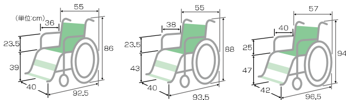
プチ NEXT-10B (低床型)
