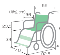
プチ NEXT-10B (低床型)
