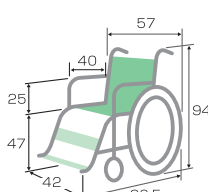
グラン NEXT-12B (高床型)
