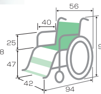
グラン NEXT-22B (高床型)
