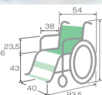
標準 NEXT-21B (標準型)
