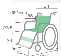
プチ NEXT-20B (低床型)
